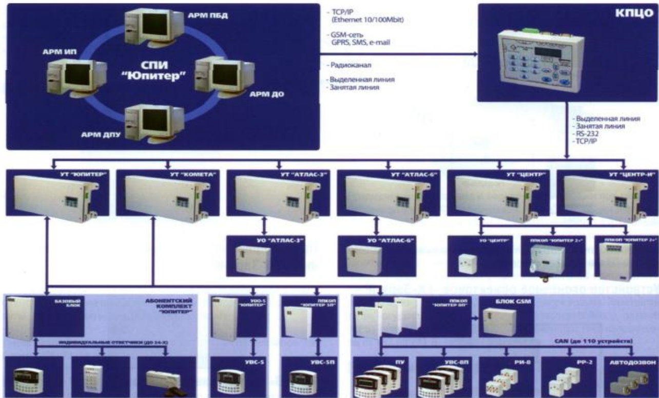
Структурная схема СПИ «Юпитер»
