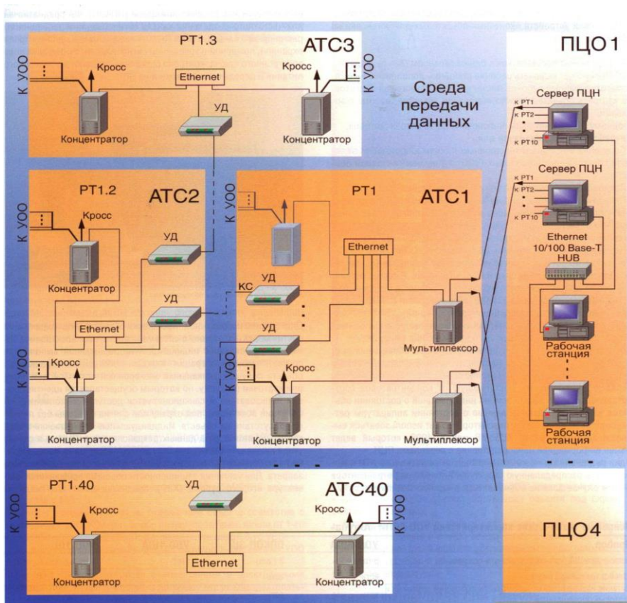
Рис. 10 – Среда передачи данных АСПИ «Ахтуба»
