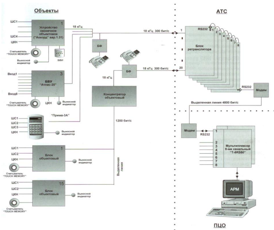
Структурная схема СПИ «Атлас-20»
