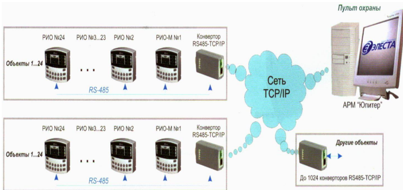
Рис.8 – Структурная схема СПИ «Юпитер»
