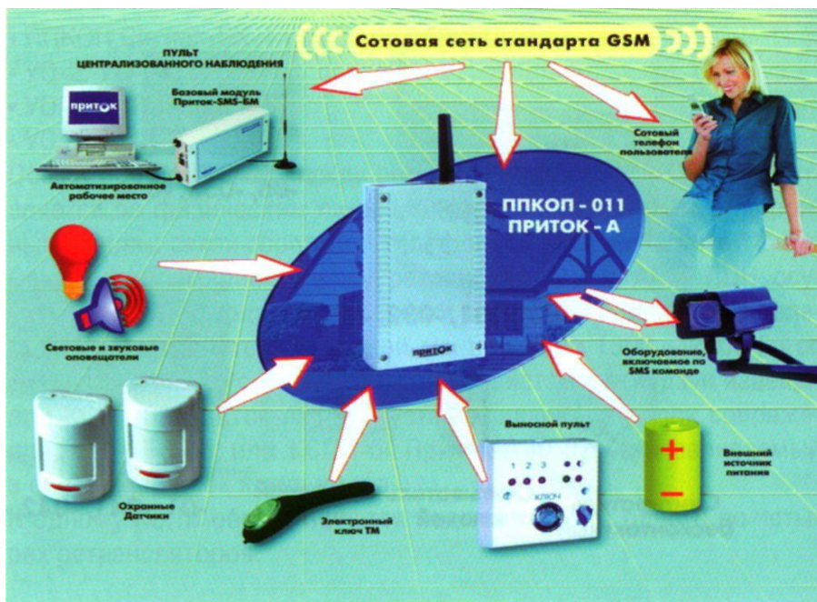
Рис.4 – Подсистема «Приток-GSM»
