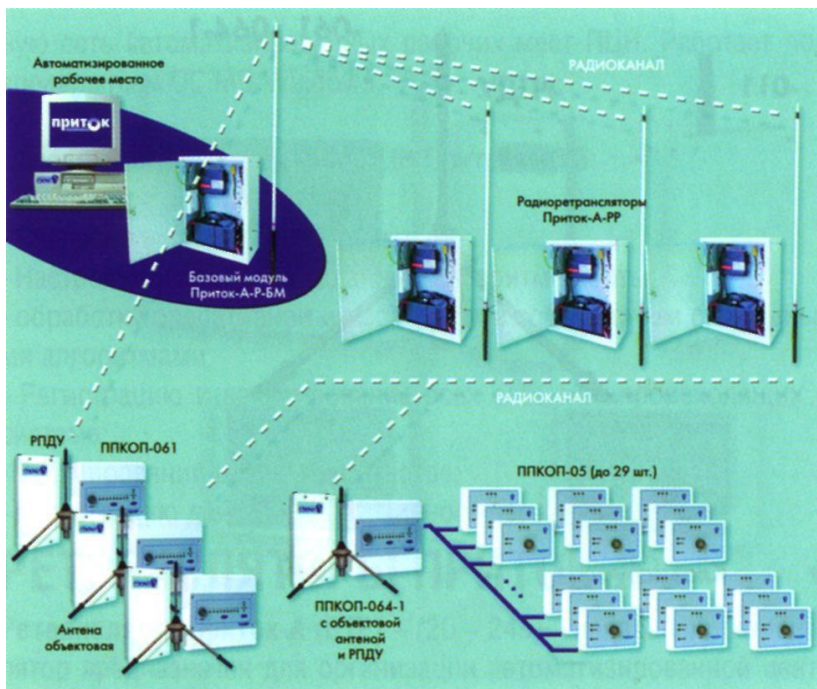
Рис.3 - Подсистема «Приток-ТСР/IP».
