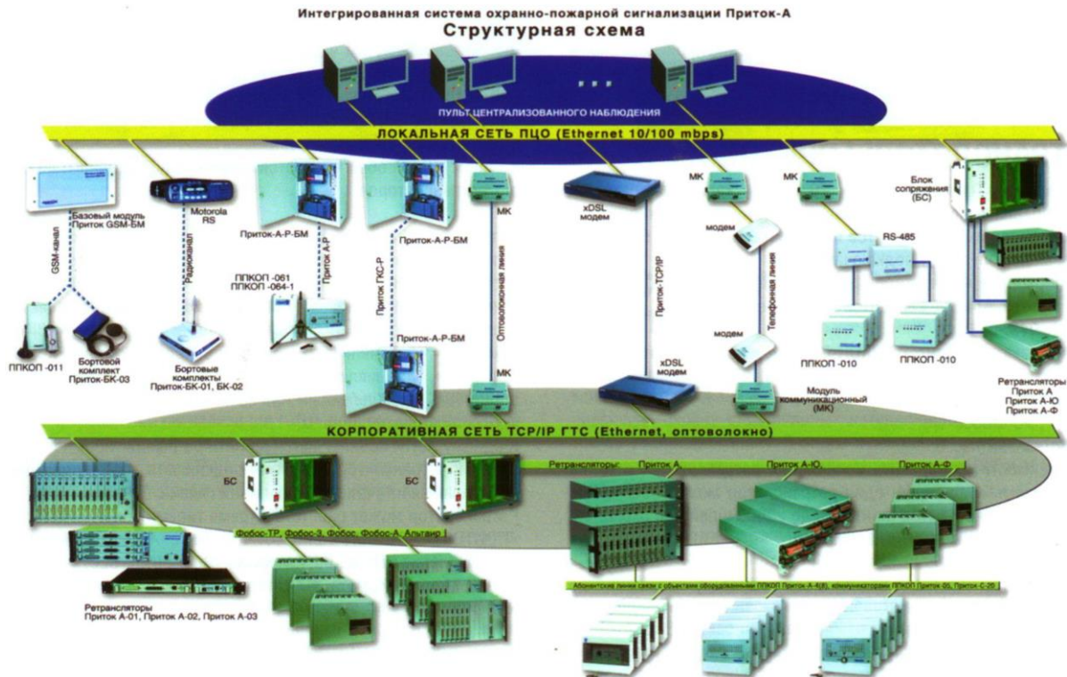
Рис. 2 – Структурная схема интегрированной системы охранно-пожарной сигнализации «Приток-А»
